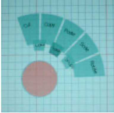
c. Submenu under "Tool" menu.
